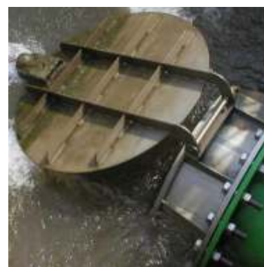
Clapet SG in acciaio inox per sezioni circolari Stainless steel flap valve for circular section
