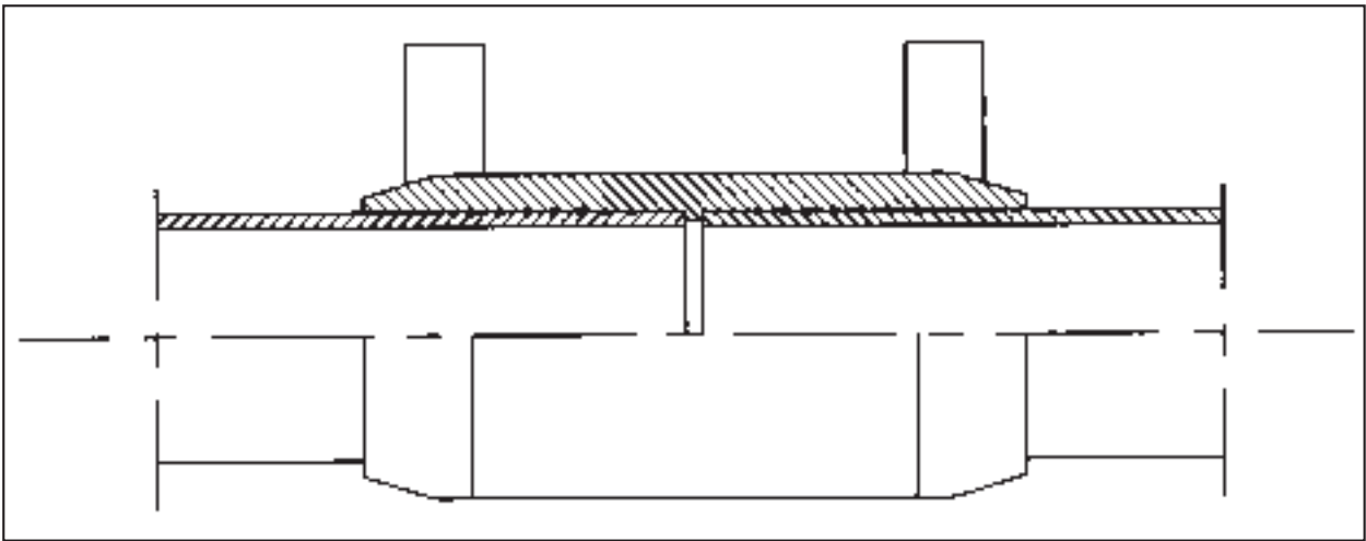
Fig. 2 - Saldatura per elettrofusione tra manicotto e tubazioni
