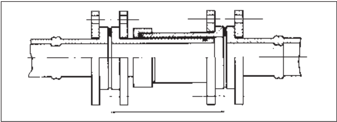
Fig. 18 - Giunto a cannocchiale
